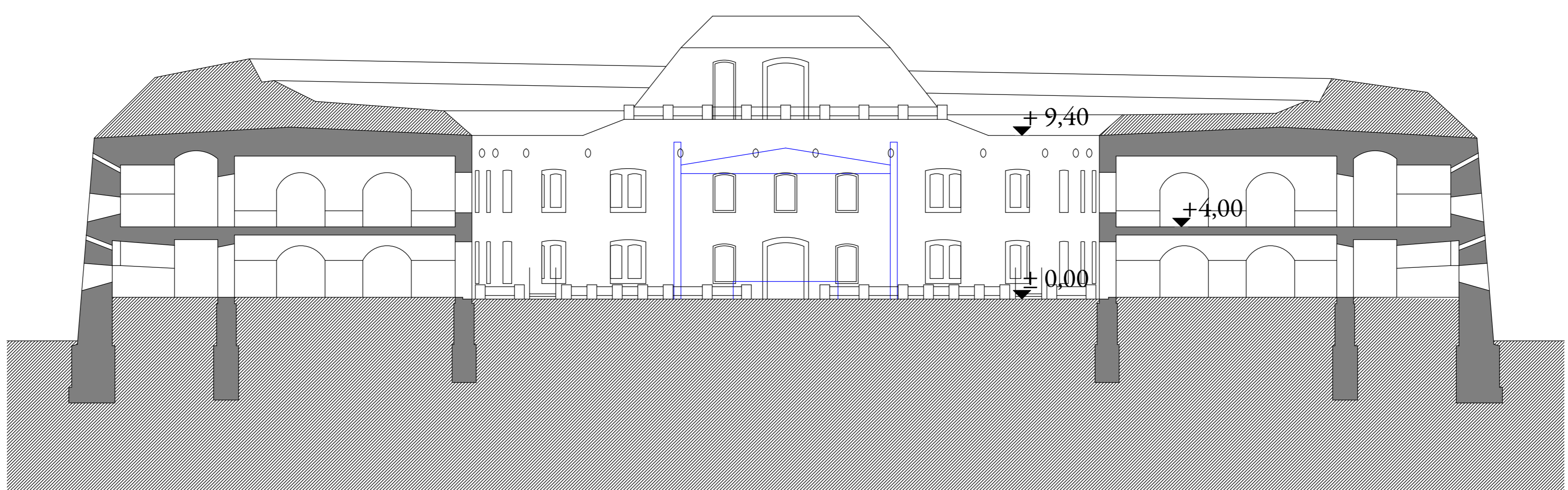
B-B METSZET
