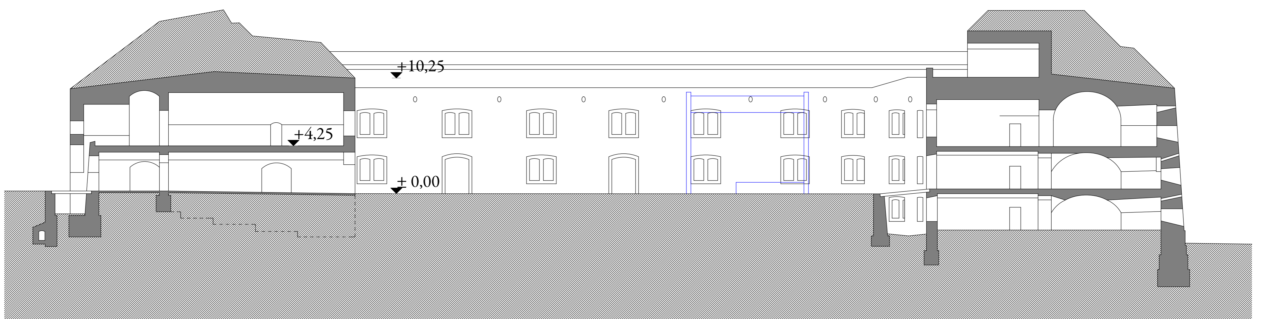
A-A METSZET
